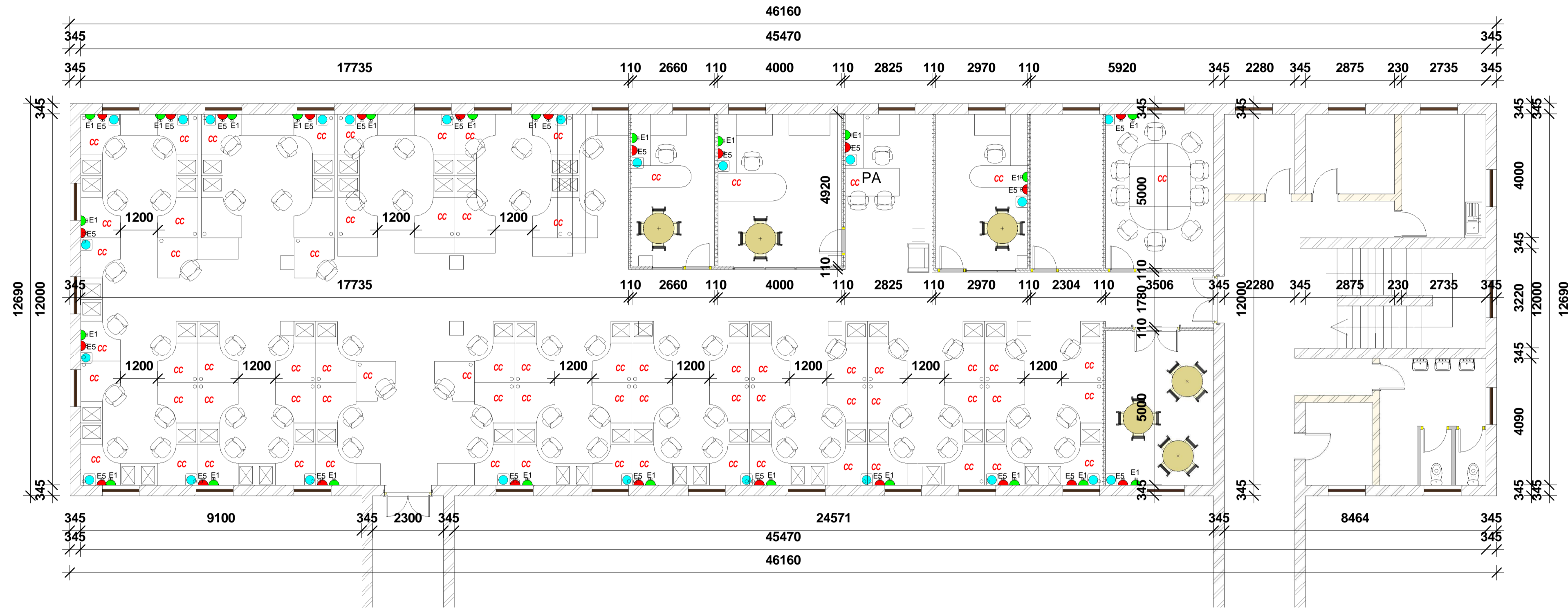
01 ELECTRICAL LAYOUT 1 : 100
